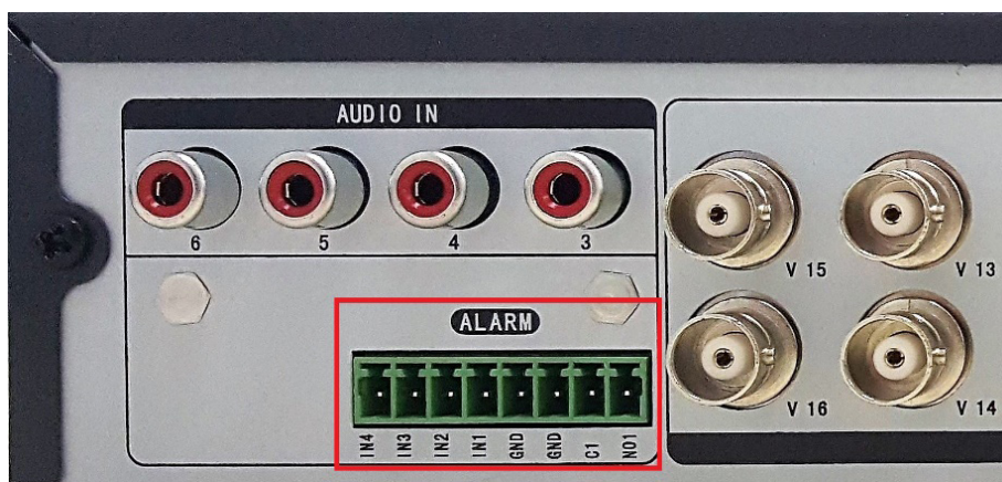
Figura 8.1.2 – I/O Allarme Mod. VS-UVR6016-LT
